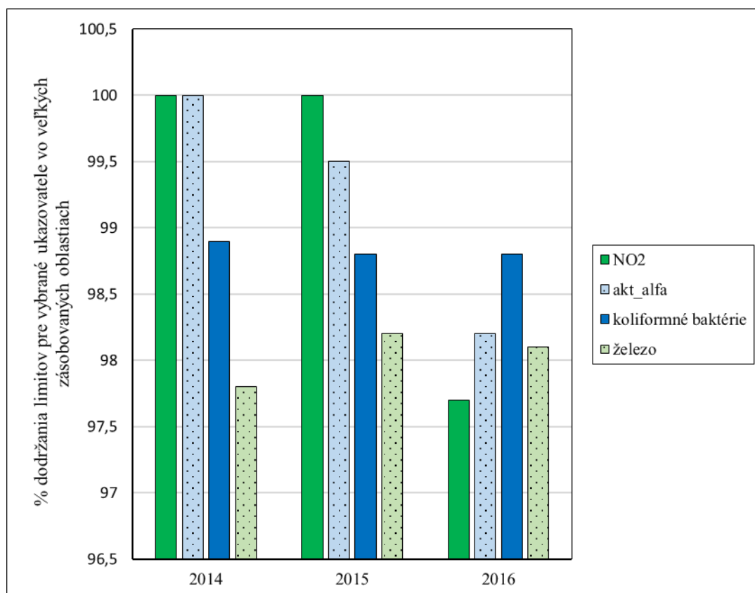
Graf č.1: Porovnanie najčastejšie prekračovaných ukazovateľov vo veľkých zásobovaných oblastiach v rokoch 2014 - 2016
